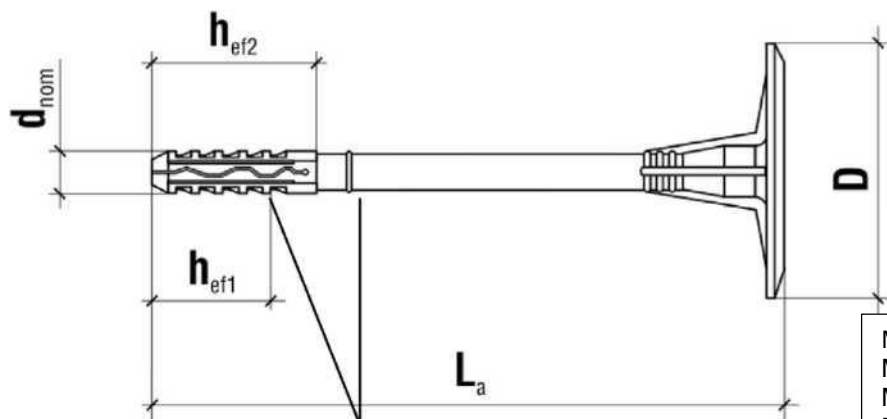
Marcaje ale adâncimii efective de ancorare
